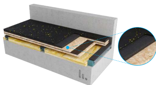
Stravigym HP avec Stravigym GympactLayer-20
